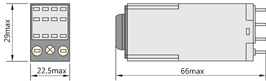
Профильные установочные размеры JSZ6
