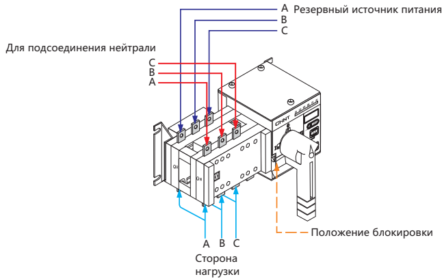
16_100A Схема трехполюсного подключения
