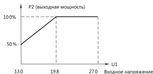
Рис. 1 Кривая выходной мощности Когда напряжение от однофазного стабилизированного источника напряжения падает ниже 198 В, выходная мощность изделия уменьшается. Изделие нужно использовать после уменьшения мощности.
