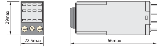
Профильные установочные размеры JSZ6
