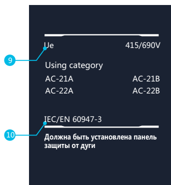
Паспортная табличка выключателя-разъединителя NXHM
