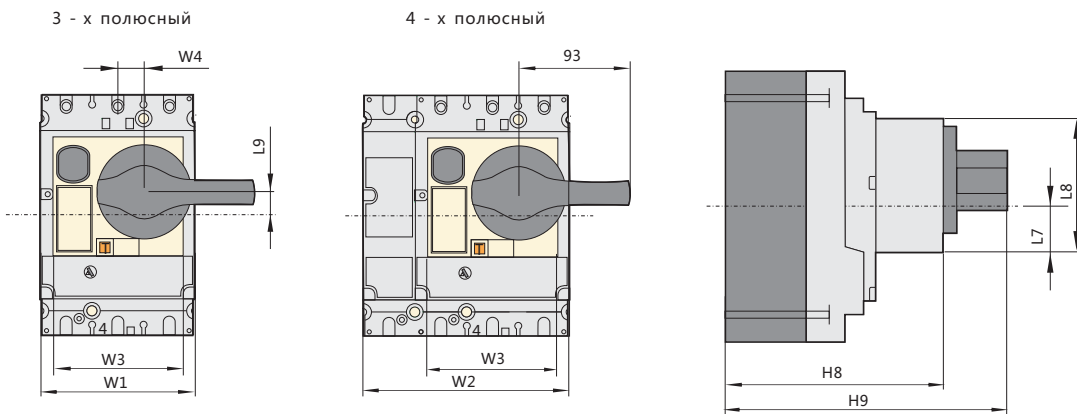
Разметка панели ( для выключателей стационарного и вычного исполнения)
