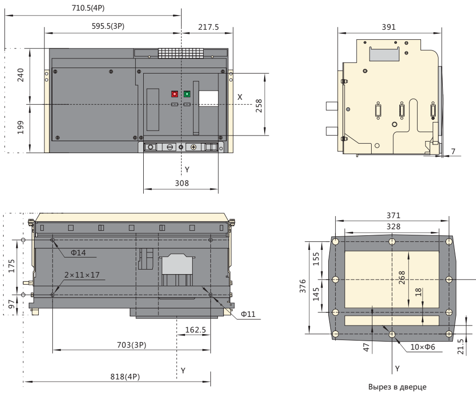
NA8G-6300 In=(6300A) выдвижное исполнение
