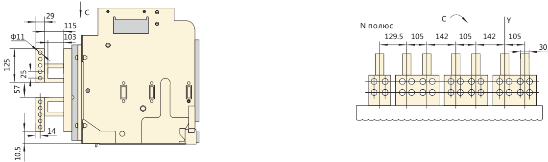
NA8G-6300( I_n=4000A\sim 5000A ) выдвижное исполнение, заднее присоединение, вертикальные контактные пластины
