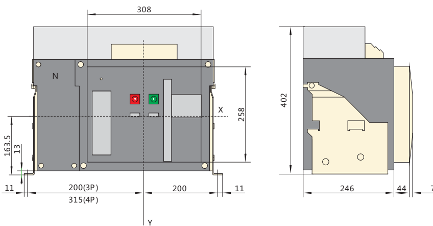
NA8G-3200 стационарное исполнение
