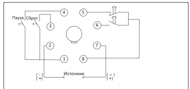
Схема соединений JSS48B
