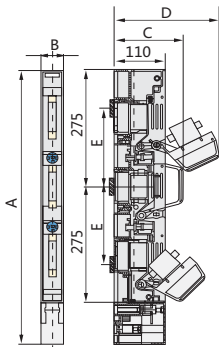
NHRT40-160 Независимое межфазное оперирование
