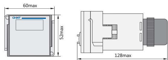
Профильные установочные размеры изделий серии JSS48B
