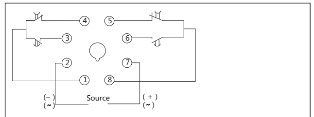
Схема соединений JSS48A-S
