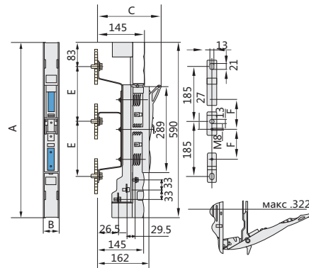
NHRT40-160/L Одновременная коммутация трех фаз
